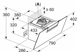
Rozmery v mm Spotrebič v režime cirkulujúceho vzduchu bez kanála
